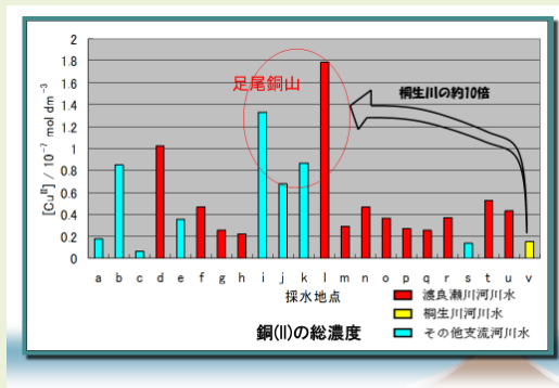
渡良瀬川水系銅 (II) 総濃度
